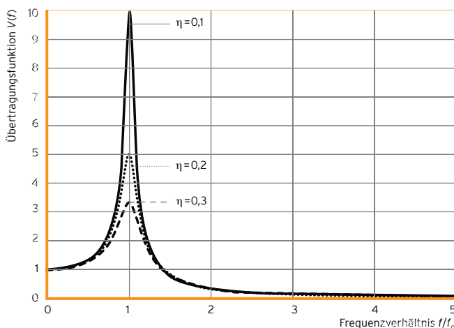
Abb. 9: Übertragungsfunktion
