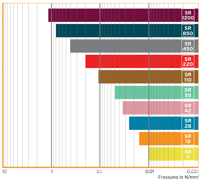
Abb. 1: Sylomer® Typenreihe
