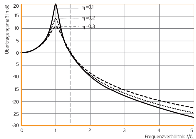
Abb. 10: Übertragungsmaß
