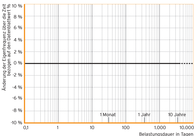
Abb. 6: Dynamisches Dauerstandverhalten von Sylomer®
